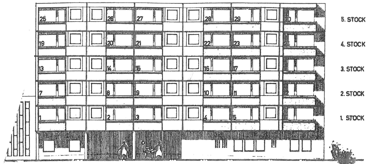
SÜDFASSADE
